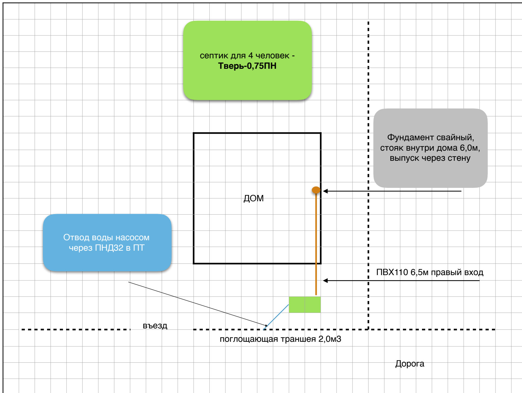
схема Тверь-0,75ПН, Первая образцовая типография, Домодедовский район
